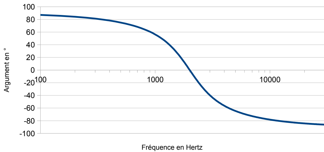
Diagramme de Bode en phase du filtre de Rauch
