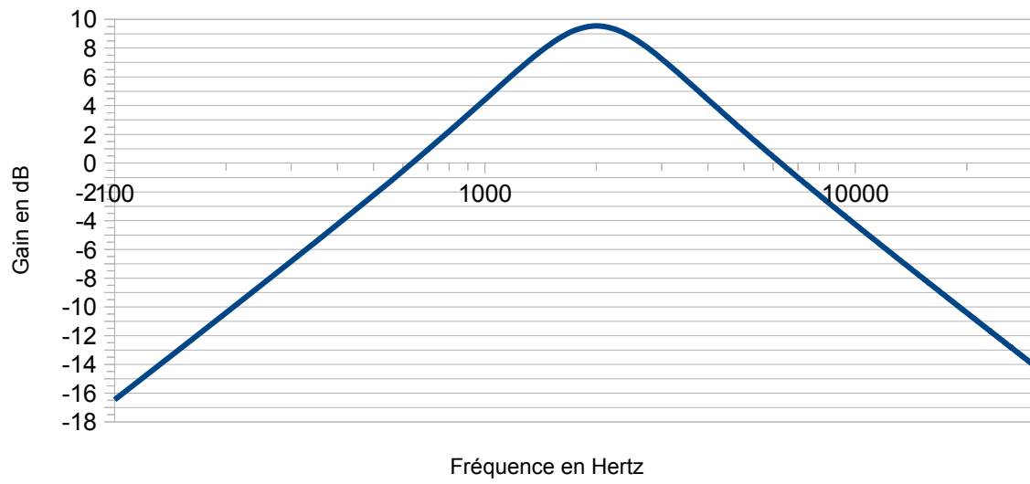
Diagramme de Bode en gain du filtre de Rauch
